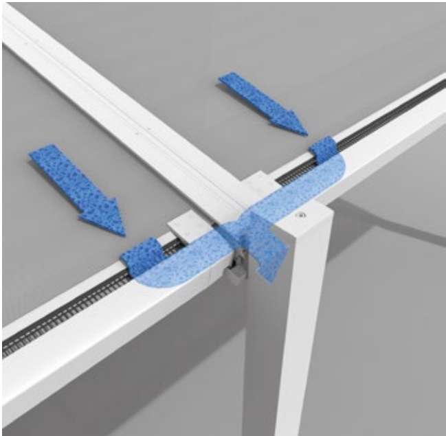
Integrált vízelvezetés
