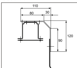
Karnis tartó konzol E50K típushoz – felső rögzítés (anyag: alumínium)
