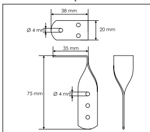
Zsinór tartó E50 típushoz
