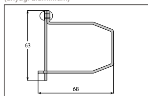
Karnis tartó konzol E50K típushoz – fali rögzítés (anyag: alumínium)
