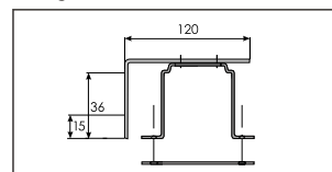
Karnis tartó konzol-2 fali rögzítéshez
