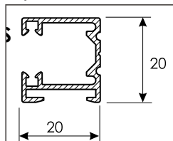
Alap vezetősín
