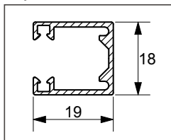
O típusú lefutósín
