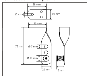
Zsinór tartó csavaros feszítéssel E50 típushoz
