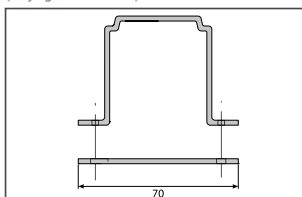
Karnis tartó konzol E50K típushoz – felső rögzítés (anyag: alumínium)
