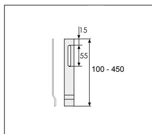
Karnis tartó konzol E50K típushoz – fali rögzítés (anyag: alumínium)
