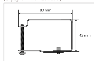
Karnis tartó konzol E50K típushoz – felső rögzítés (anyag: cink borítású acél)
